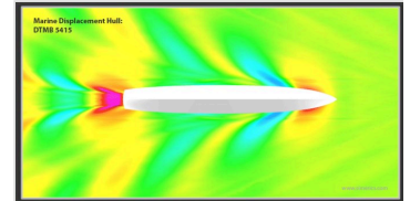
Carène à déplacement DTMB 5415
